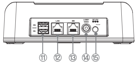
제품의 뒷면
